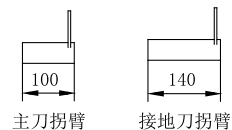
主刀拐臂
